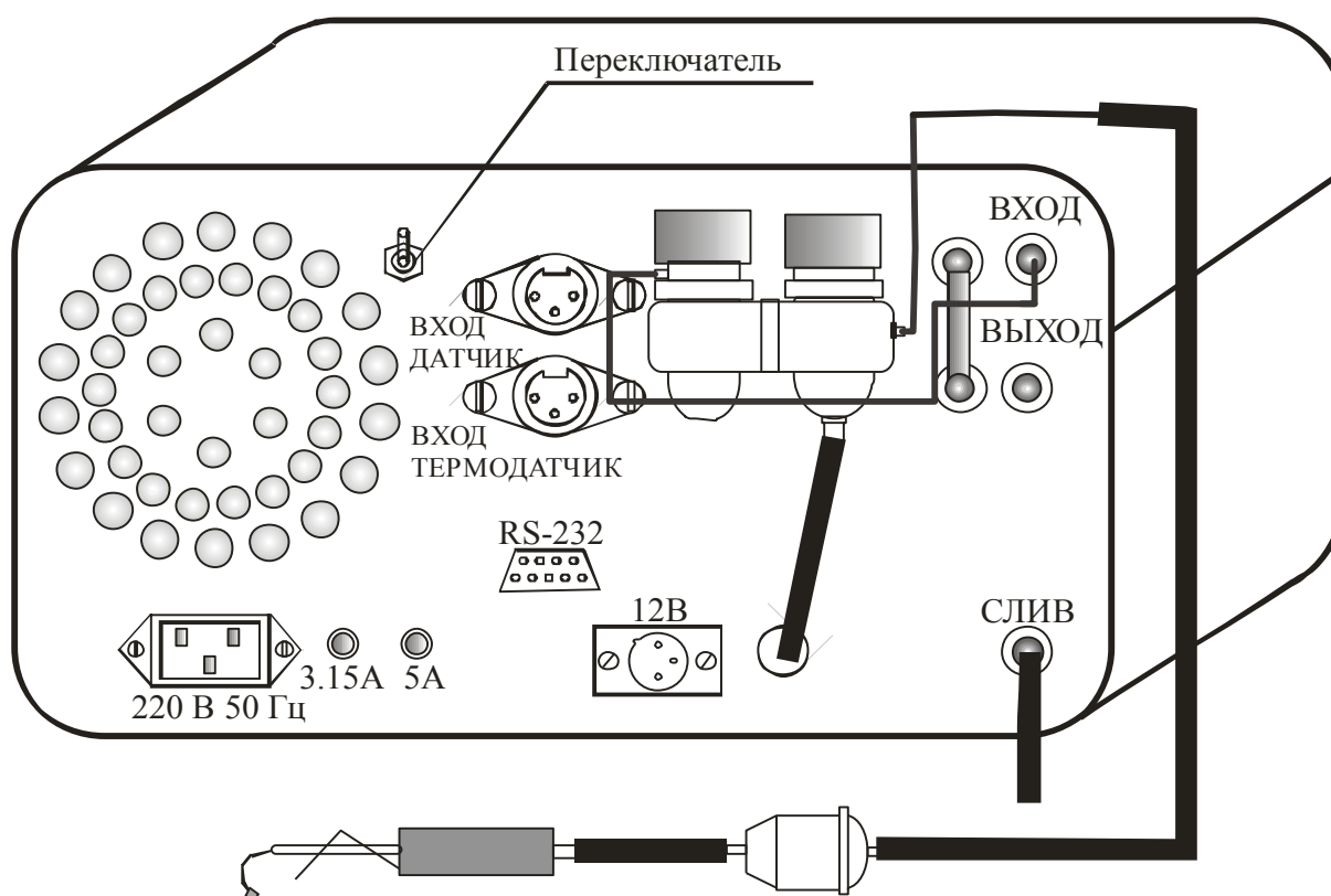
Рис.5 Схема пробоотбора
