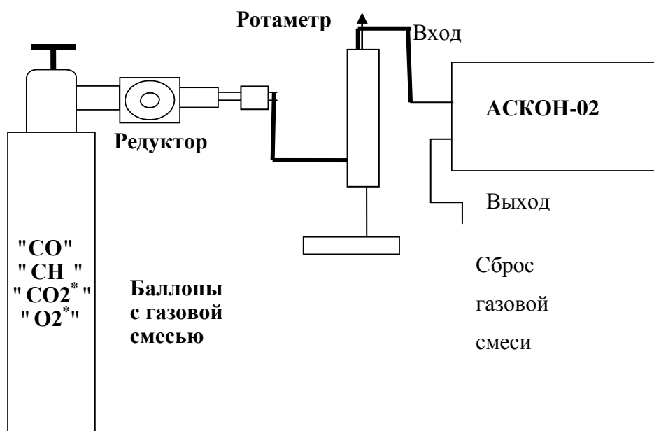
Рисунок 6 Пневмосхема для поверки прибора
